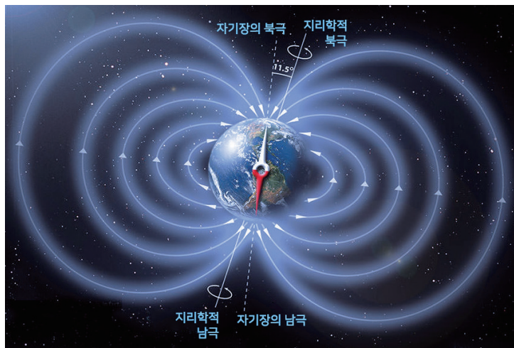
▶ 거대한 자석과도 같은 지구는 북극이 N극, 남극이 S극과 같다. 위의 그림은 지구에 의해 생성된 보이지 않는 자기장 선을 도식화했다. 이 자기장은 지구에 도달하는 우주방사선을 막아 생명이 살 수 있게 한다(출처: Peter Reid, University of Edinburgh)
